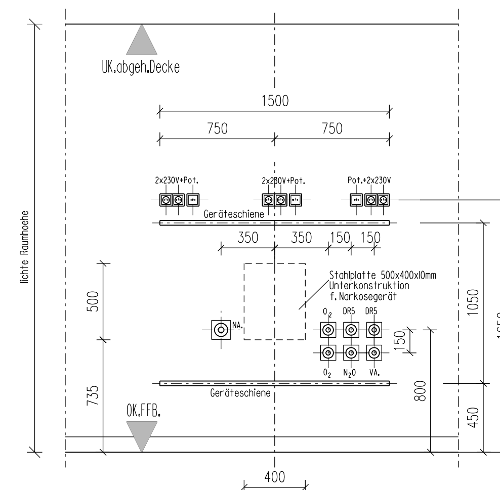
Wandansicht: Anästhesie-Arbeitsplatz (M 1:25)
